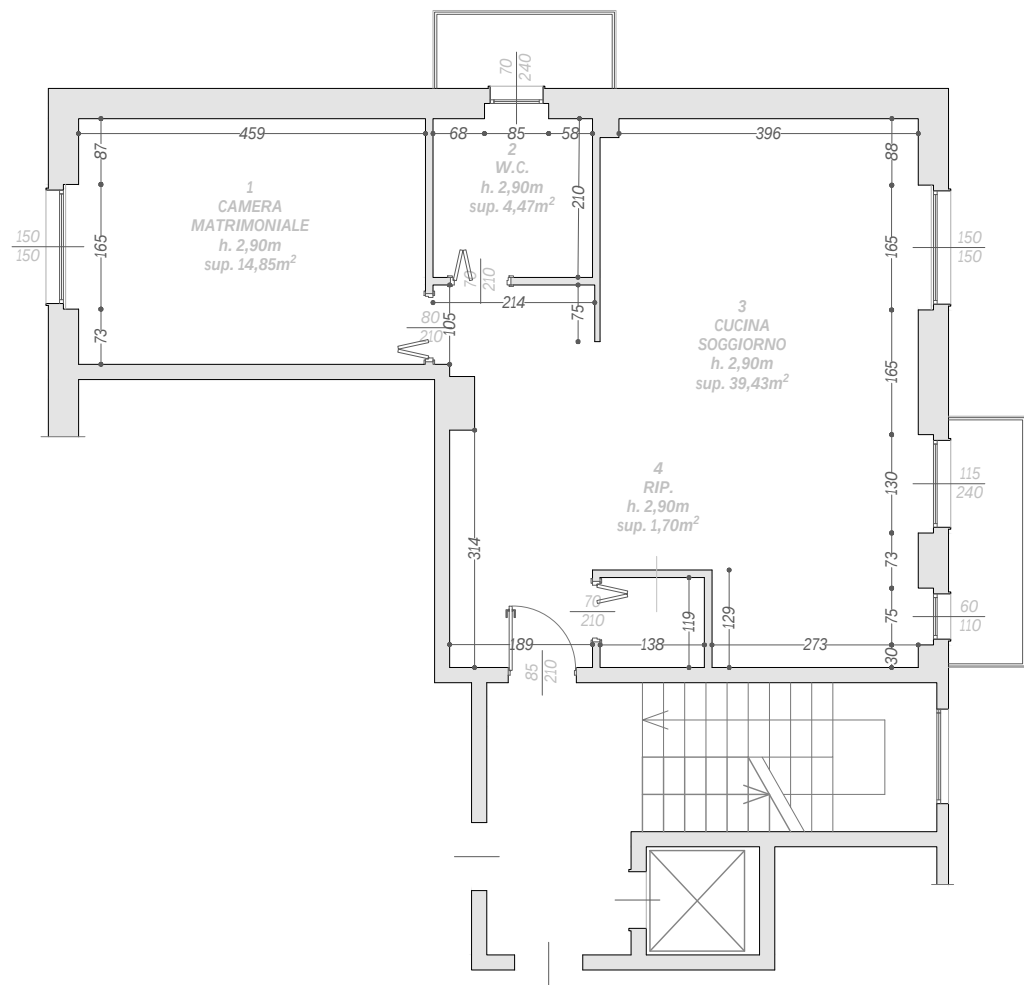
PIANTA PIANO SETTIMO - Stato di Fatto_sc 1:100
