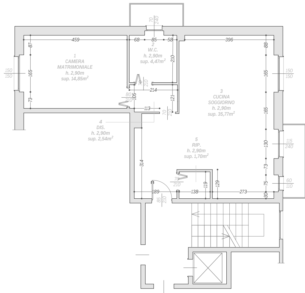
PIANTA PIANO SETTIMO - Stato di Progetto_sc 1:100
